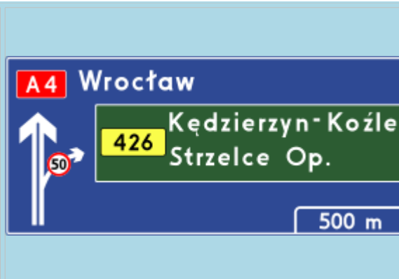
E-1a: tablica przeddrogowskazowa na autostradzie
